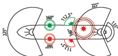
Схема расположения огней, имеет ход относительно воды
