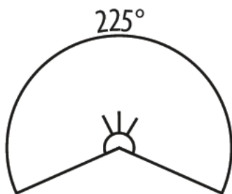
топовый огонь (Правило 21 (а), стр. 47)
