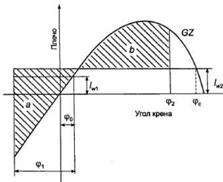
Рис.2.3.1. Воздействие сильного ветра и бортовой качки
