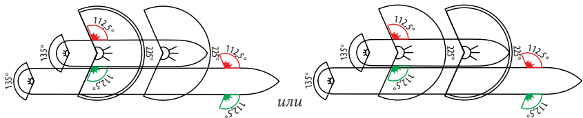
Возможные схемы расположения огней
