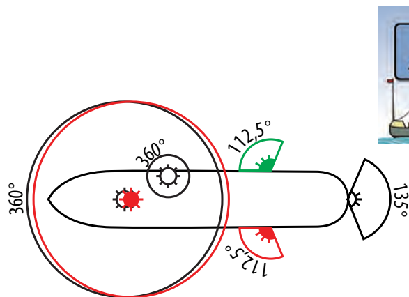
Схема расположения огней, имеет ход относительно воды
